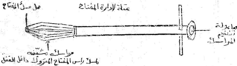
شكل يمثل : عتلة دفع المفتاح المتروك داخل القفل من الداخل
