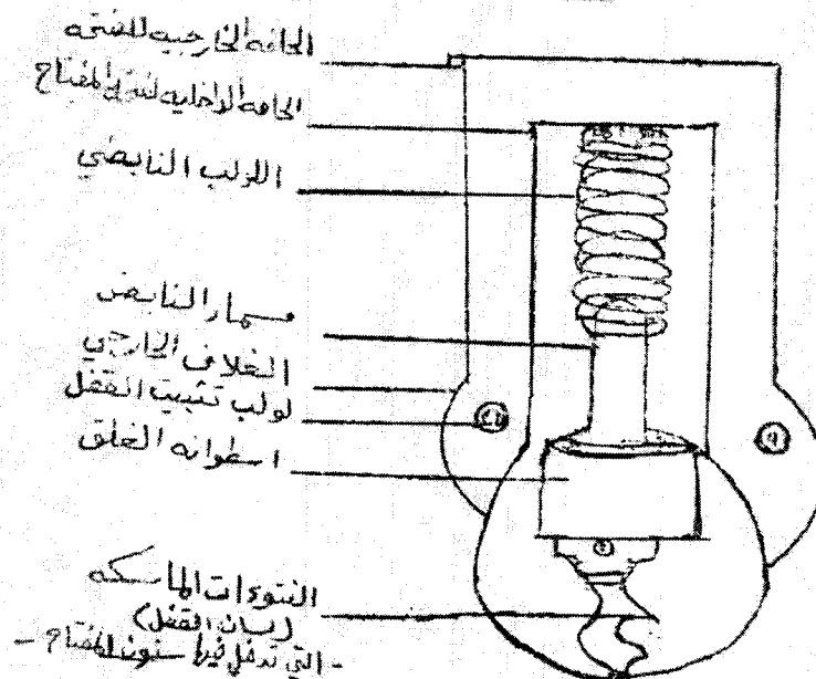
شكل يمثل مقطع عرضي لآلية قفل اعتيادي
